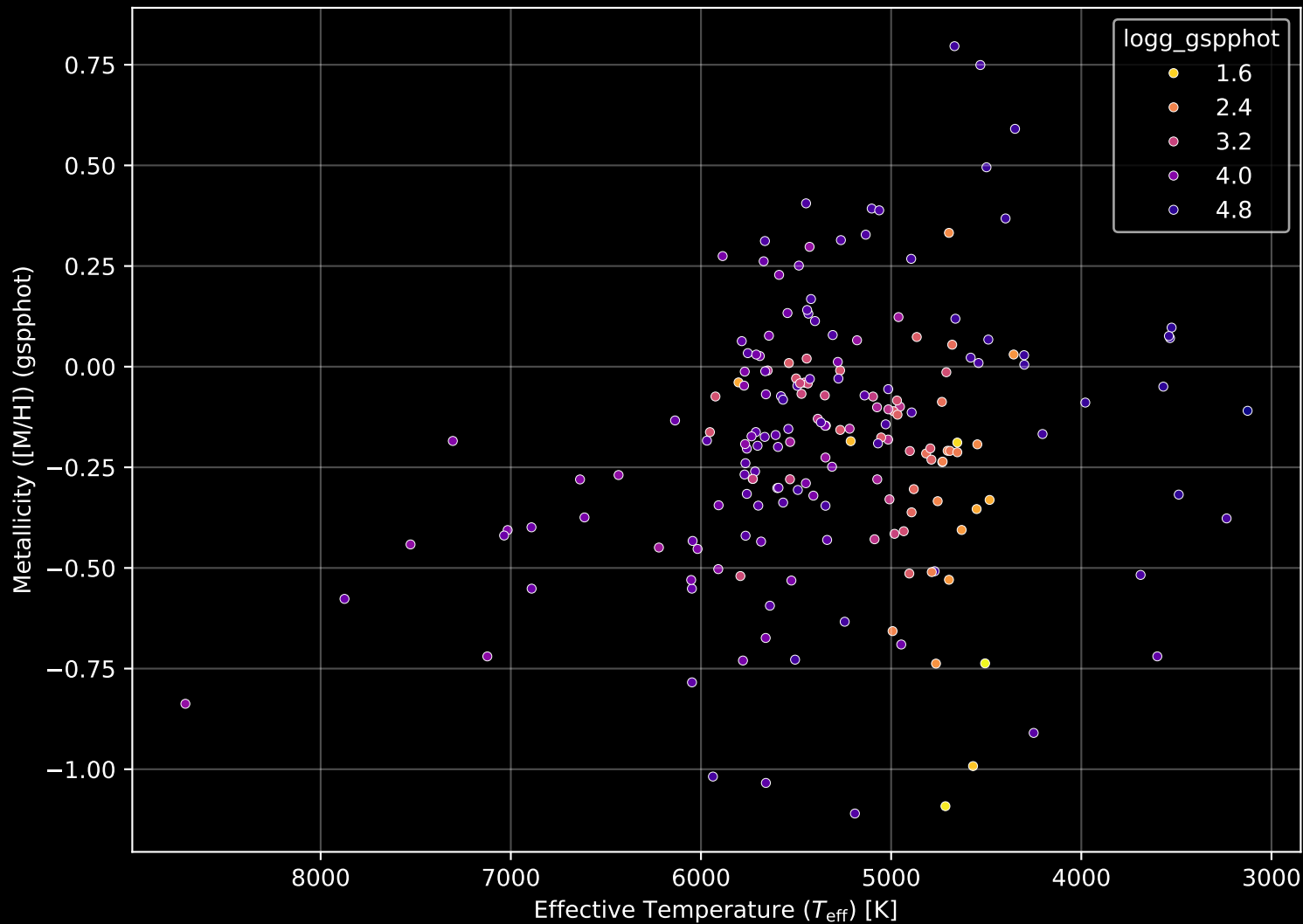
APOGEE DR17 Field: [016+48_MGA] Stellar Population Parameters (n= 192)
